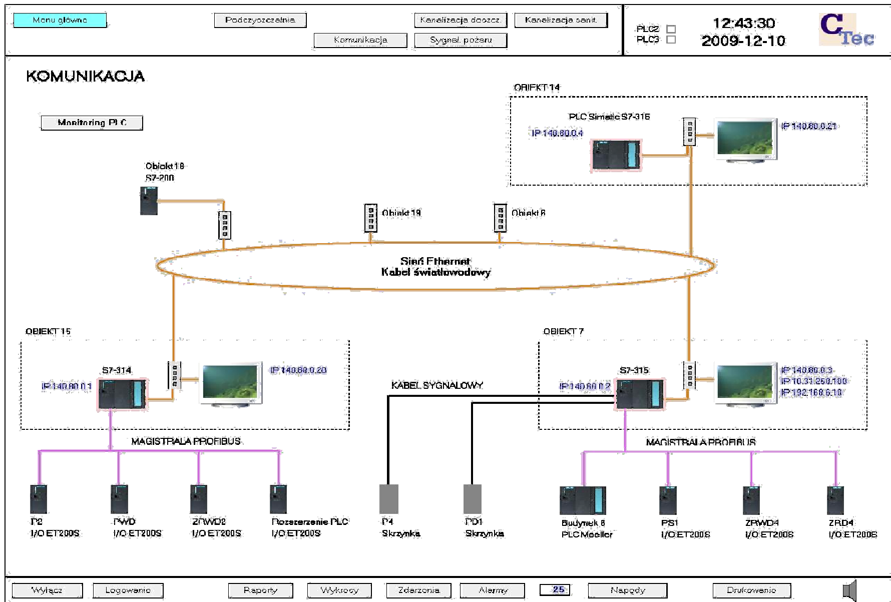
Schemat – stan istniejący AKPIA
